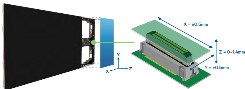
LED 模組： X、Y、Z 方向調整
